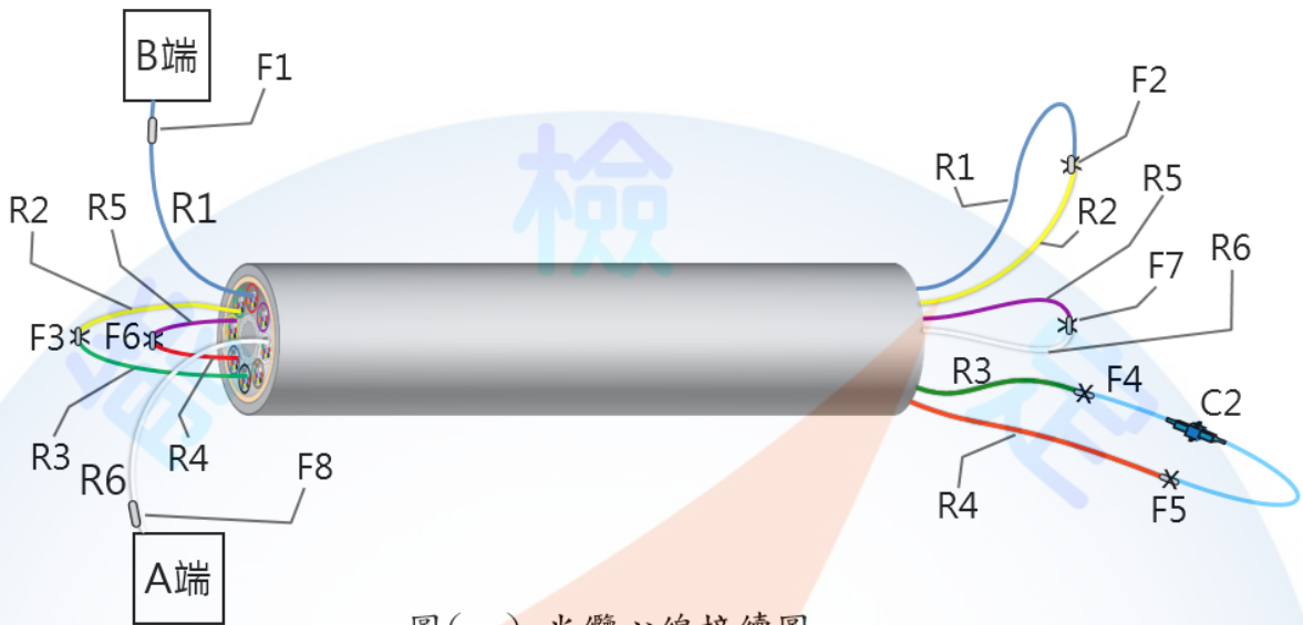
圖(一) 光纜心線接續圖
