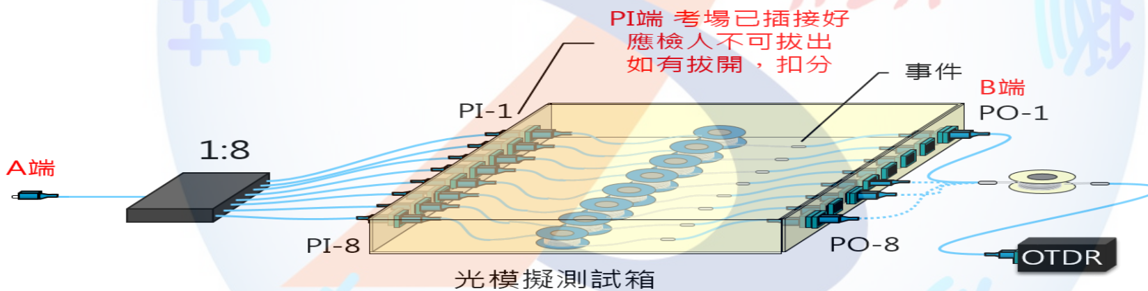
圖(3)反向掃描測試箱
