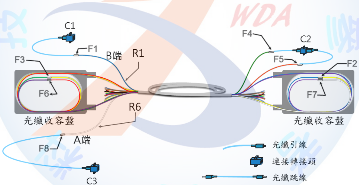
圖(二) 光纜心線鏈結收容圖
