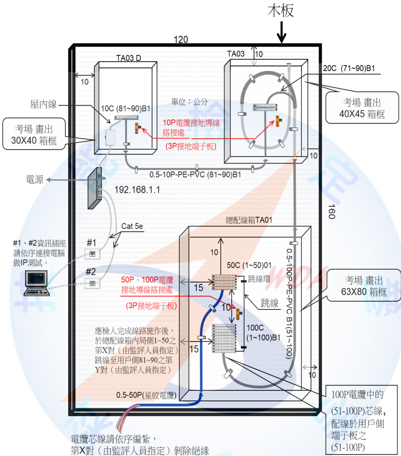
電信總配線箱、主配線箱、支配線箱纜線配接示意圖
