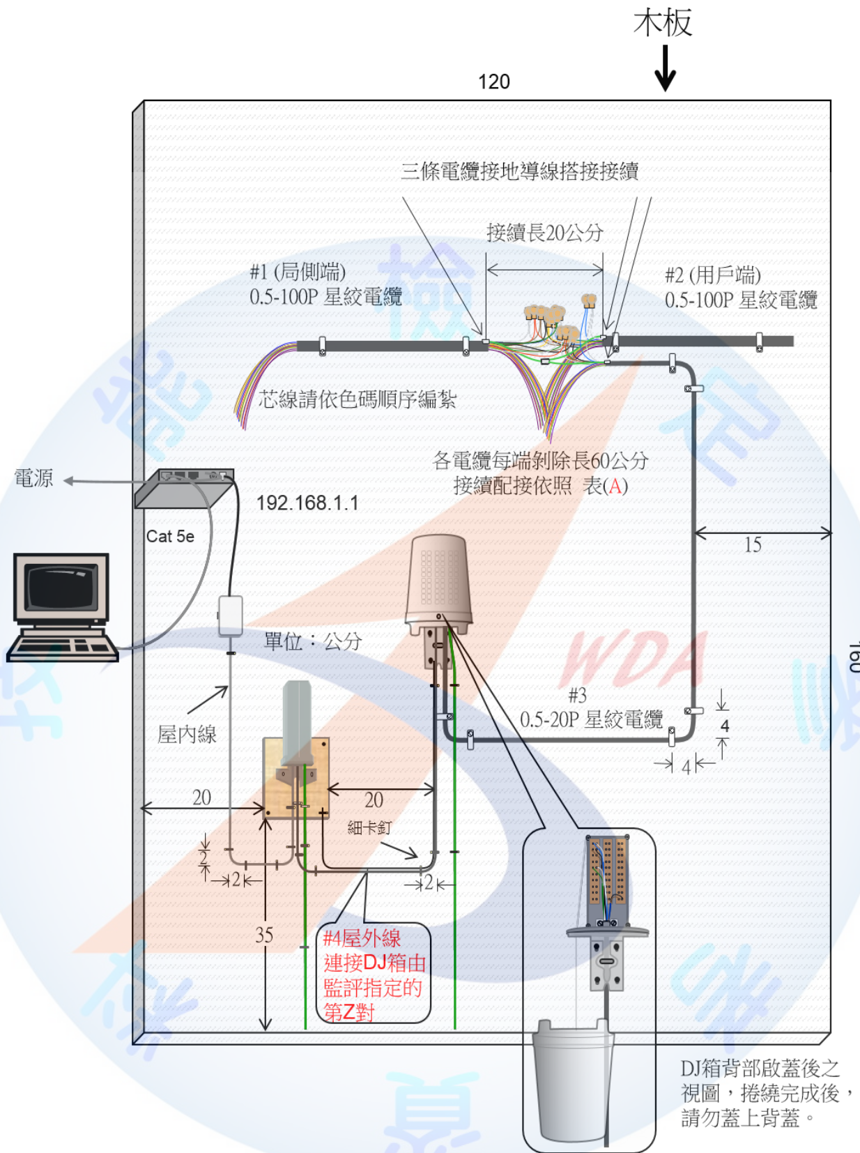
金屬電纜、DJ 箱裝接示意圖
