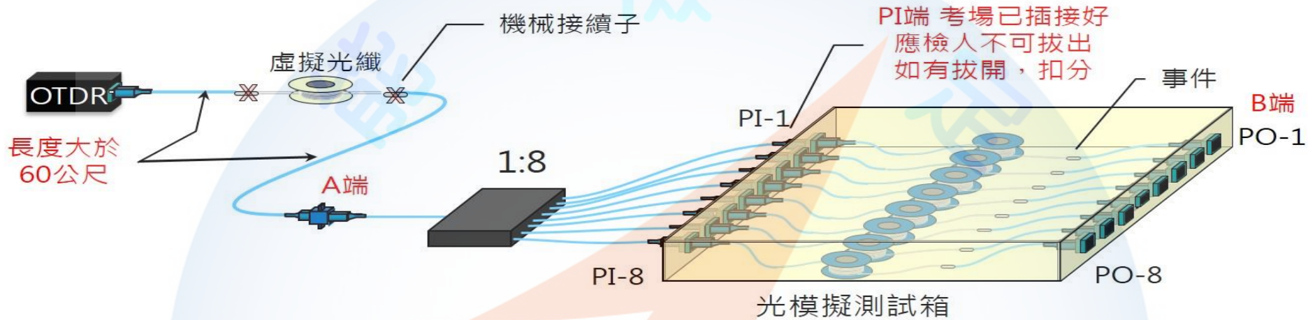
圖(2)正向掃描測試箱
