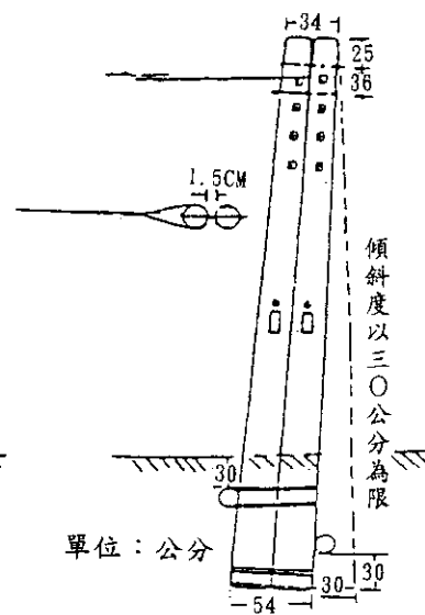
圖6-3 終端桿
