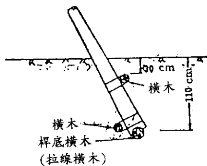
鬆軟土質及受強張力桿為防止 電桿被往上拔起裝設橫木情況
