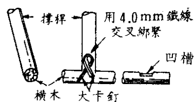
第5-45圖 撐桿橫木部裝設法
