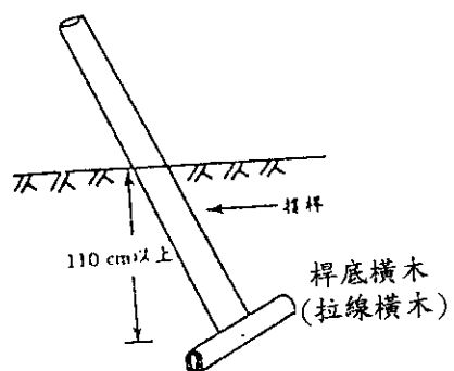
曲線桿及終端桿之撐桿裝設橫木
