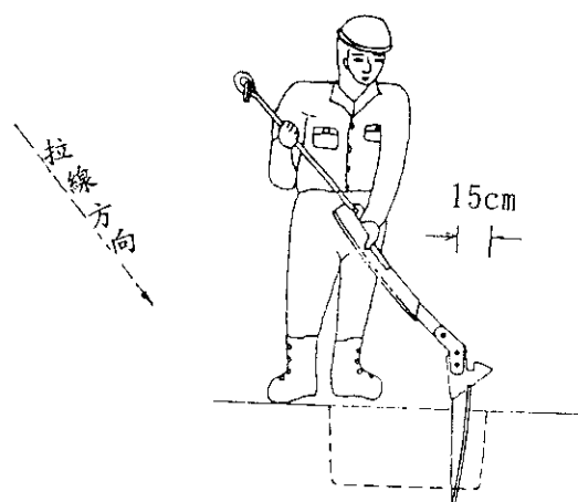
第5-11圖 抗拉板的打入①
