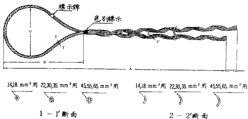
第3-6圖 1號電桿型號線夾
