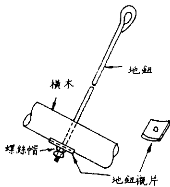
第5-8圖 地鉤裝法
