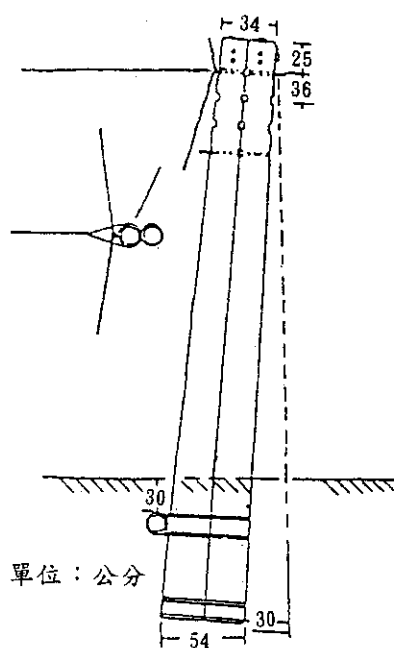
圖6-2 分岐桿
