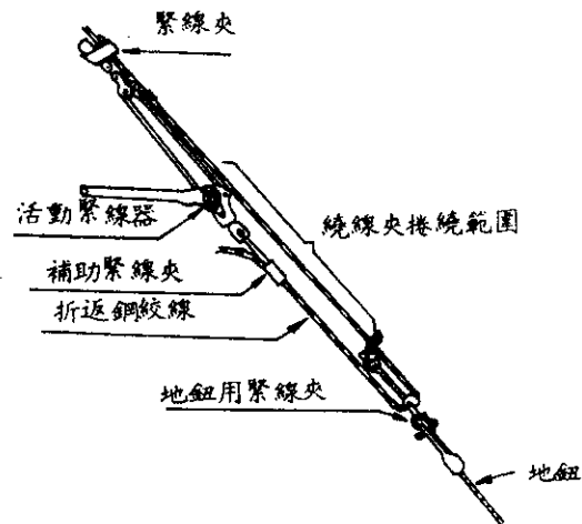
第5-37圖 緊線方法（其四）
