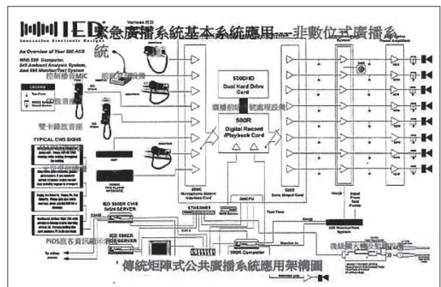
圖-1 傳統矩陣式緊急廣播系統架構圖
