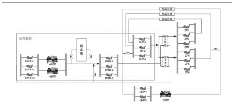
圖2.2 改善前空調冰水系統流程圖
