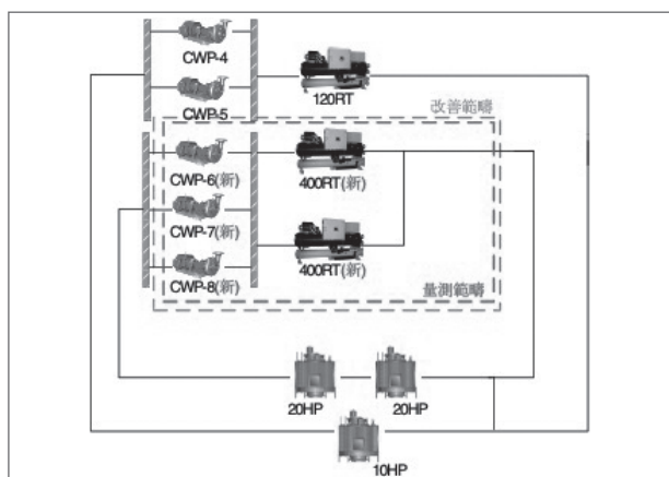
圖2.3 改善前空調冷卻水系統流程圖
