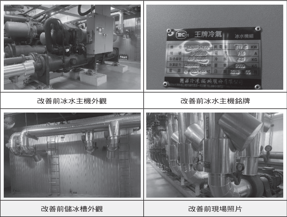
圖2.1 空調系統設備規格照片、現場照片
